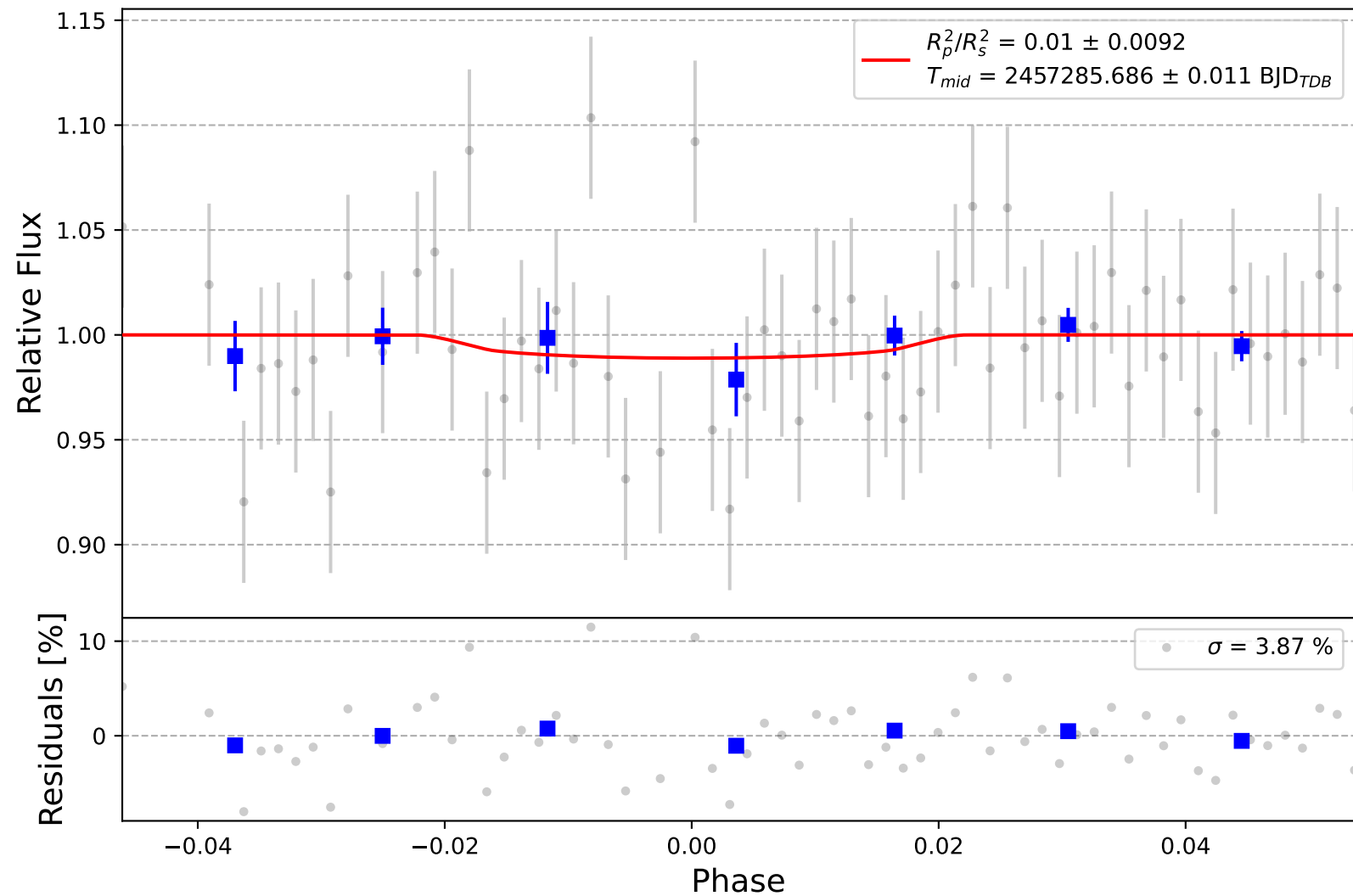
TrES-5 b
