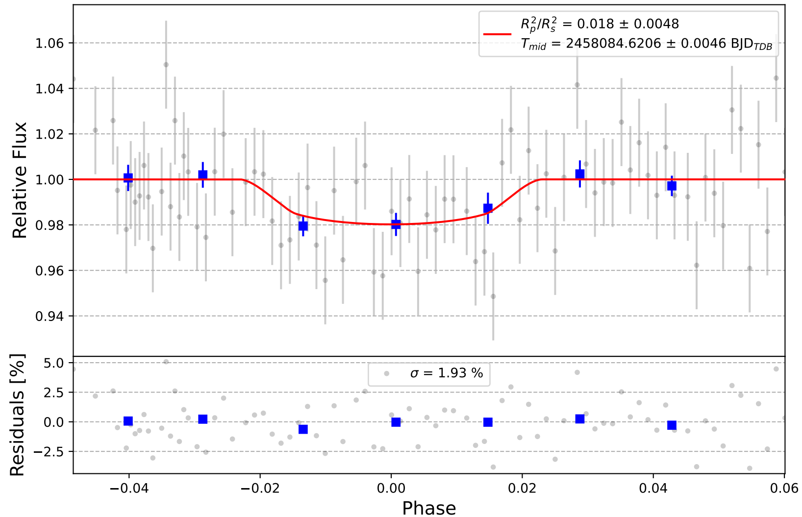
TrES-5 b
