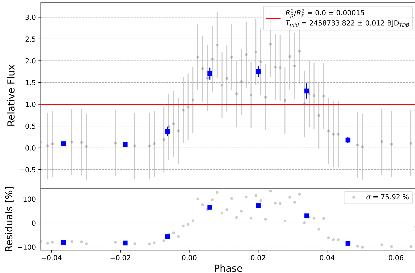
TrES-5 b
