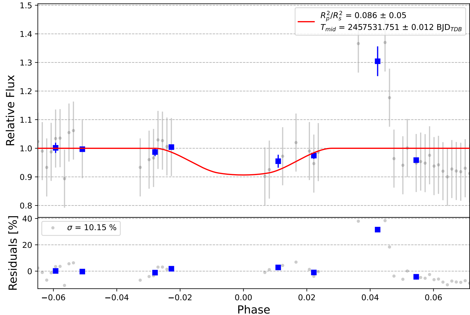
TrES-5 b
