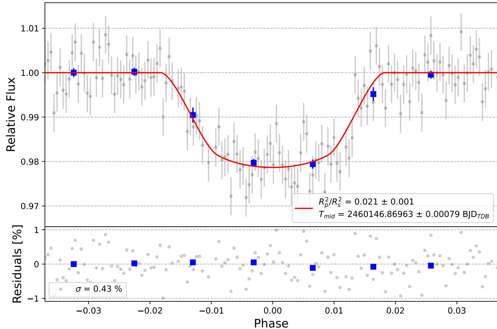
WASP-2 b
