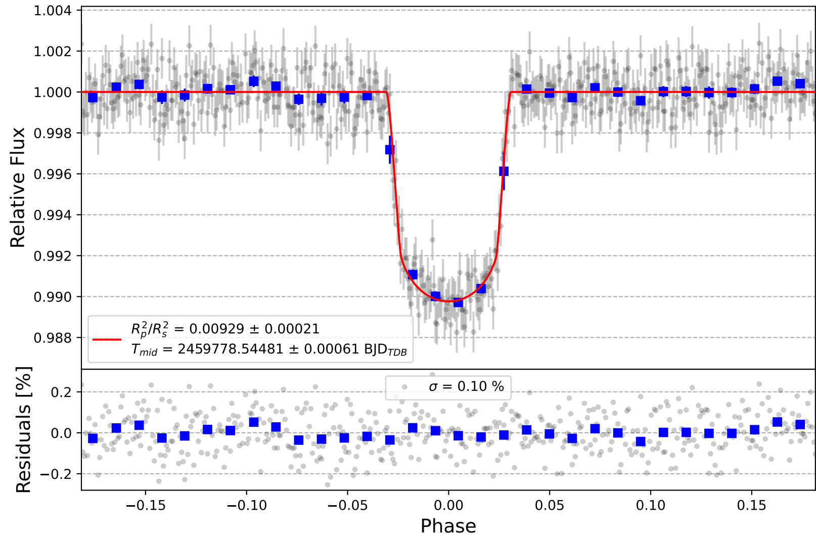
WASP-3 b
