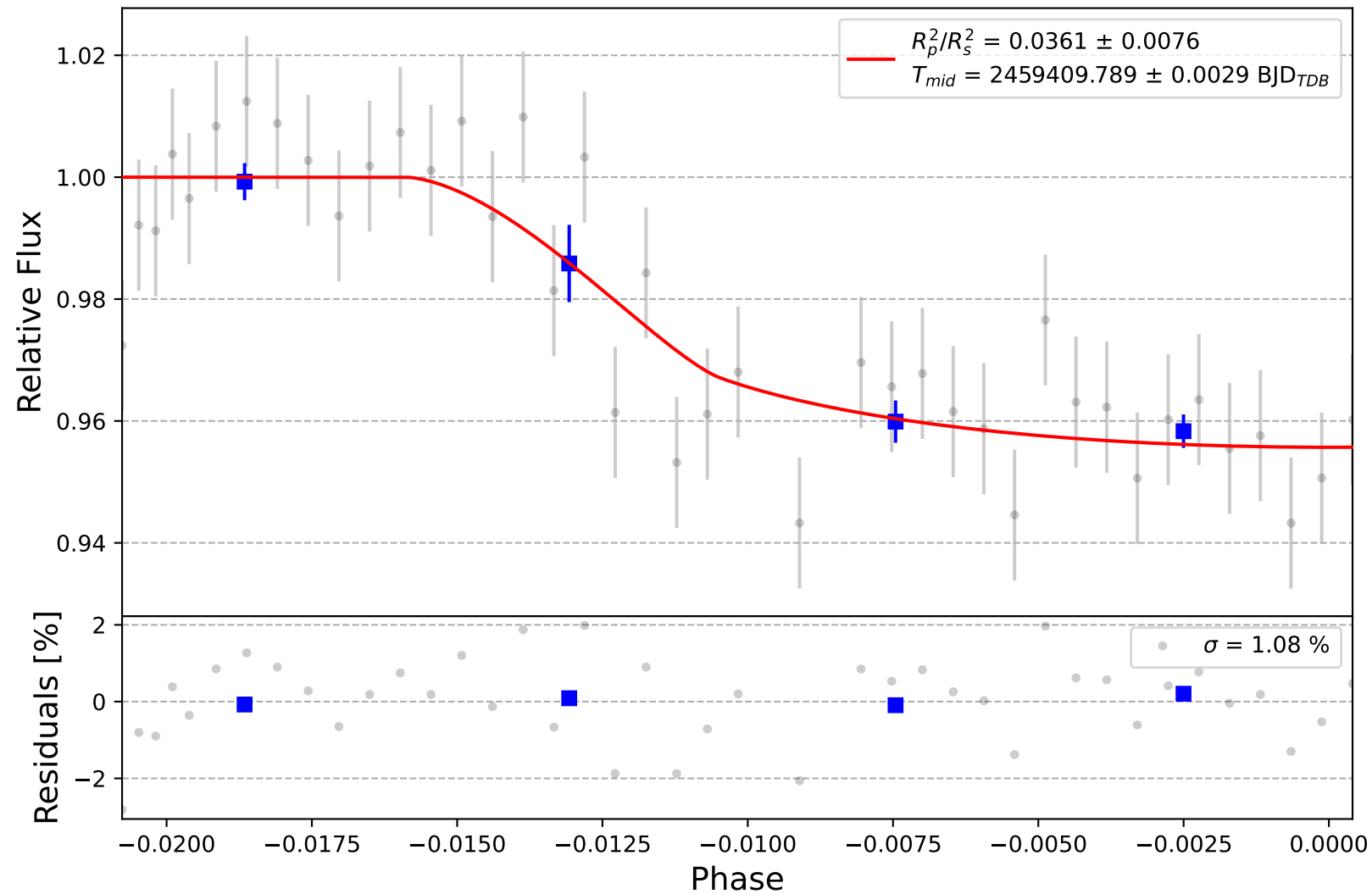
XO-1 b
