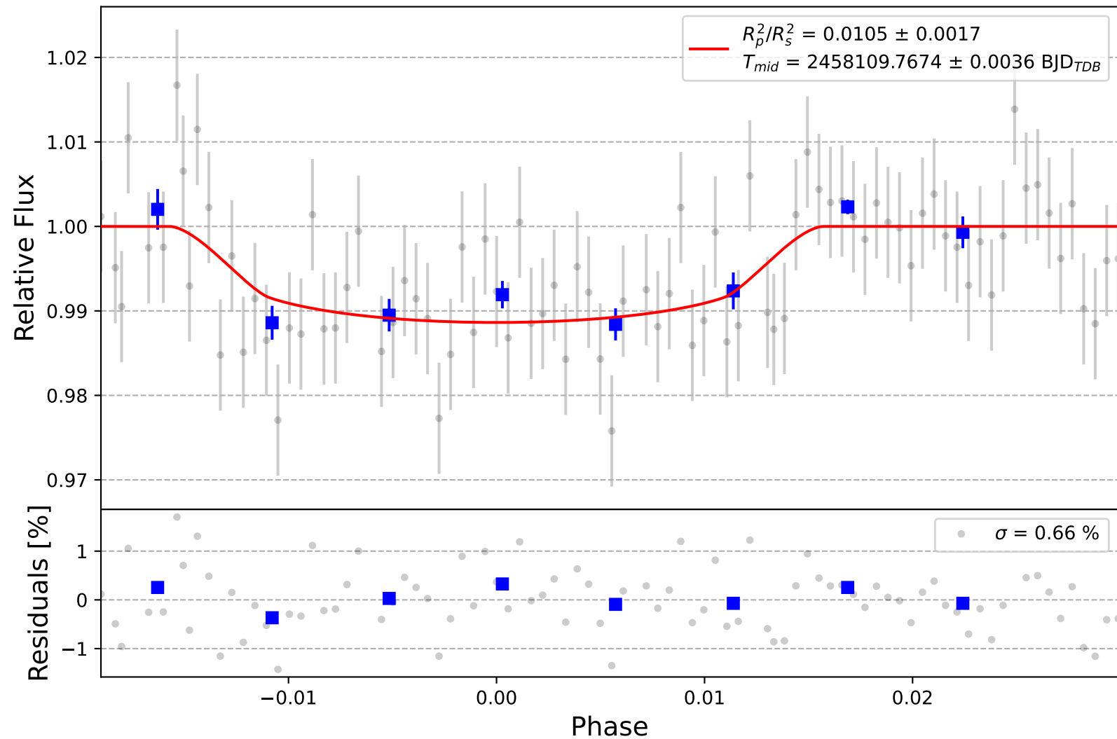
XO-6 b
