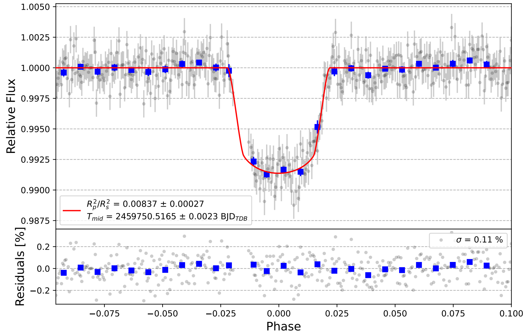
XO-7 b
