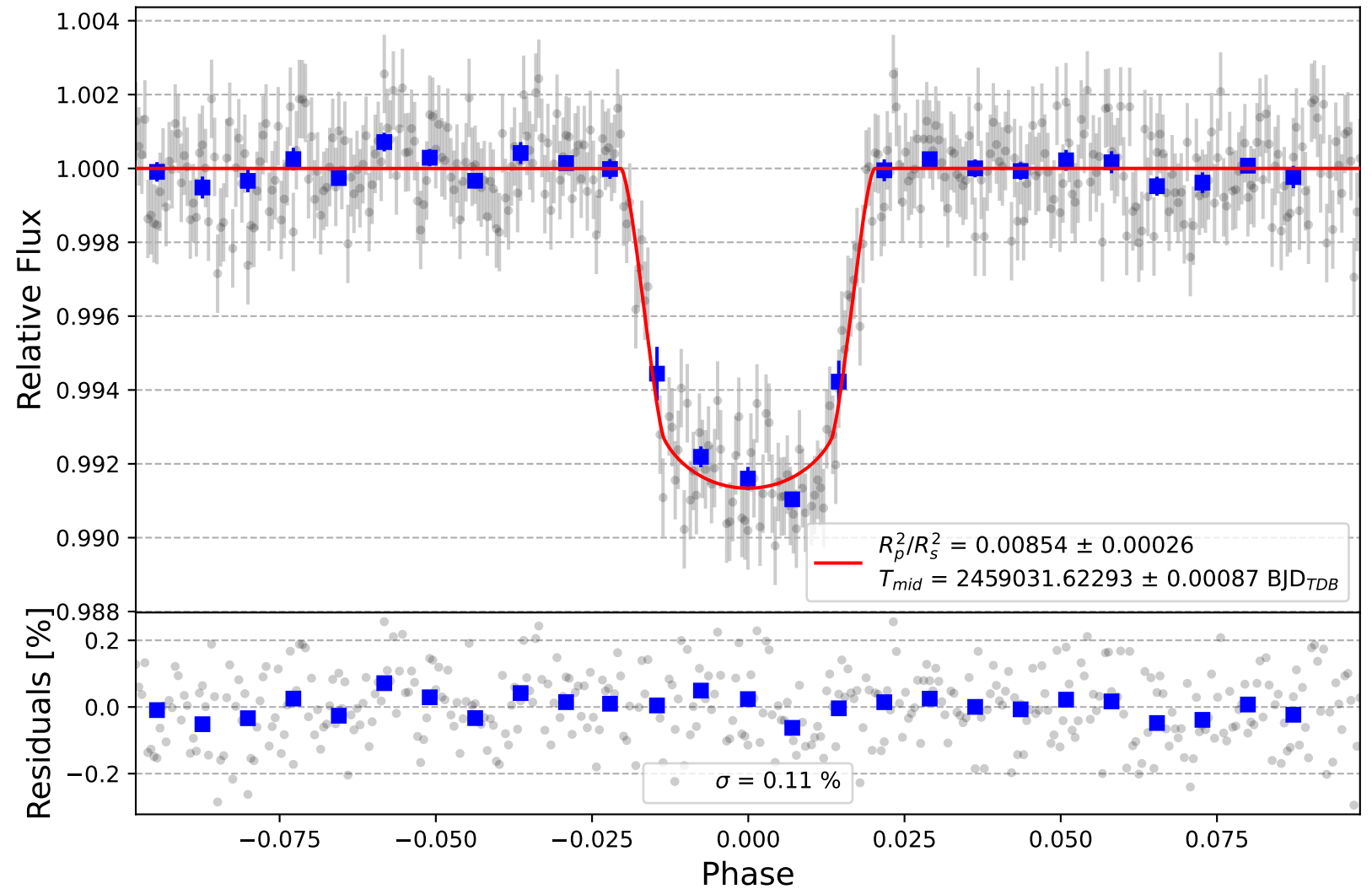
XO-7 b
