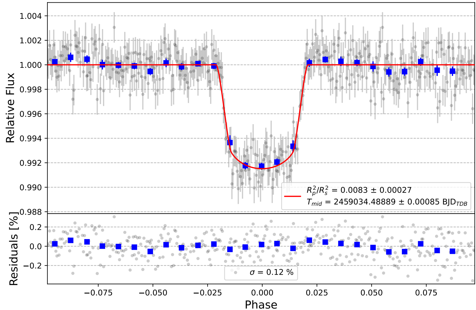
XO-7 b
