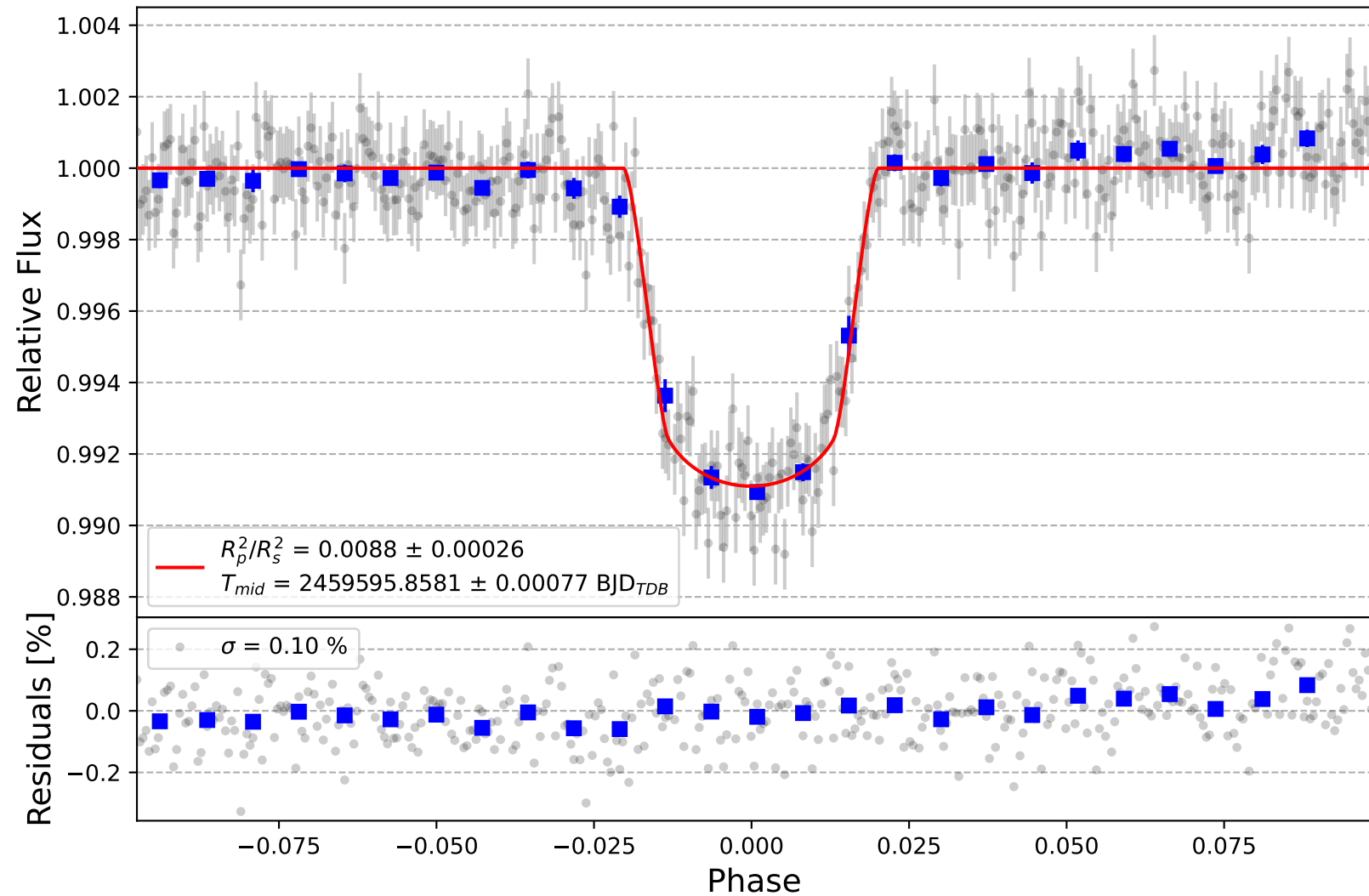
XO-7 b
